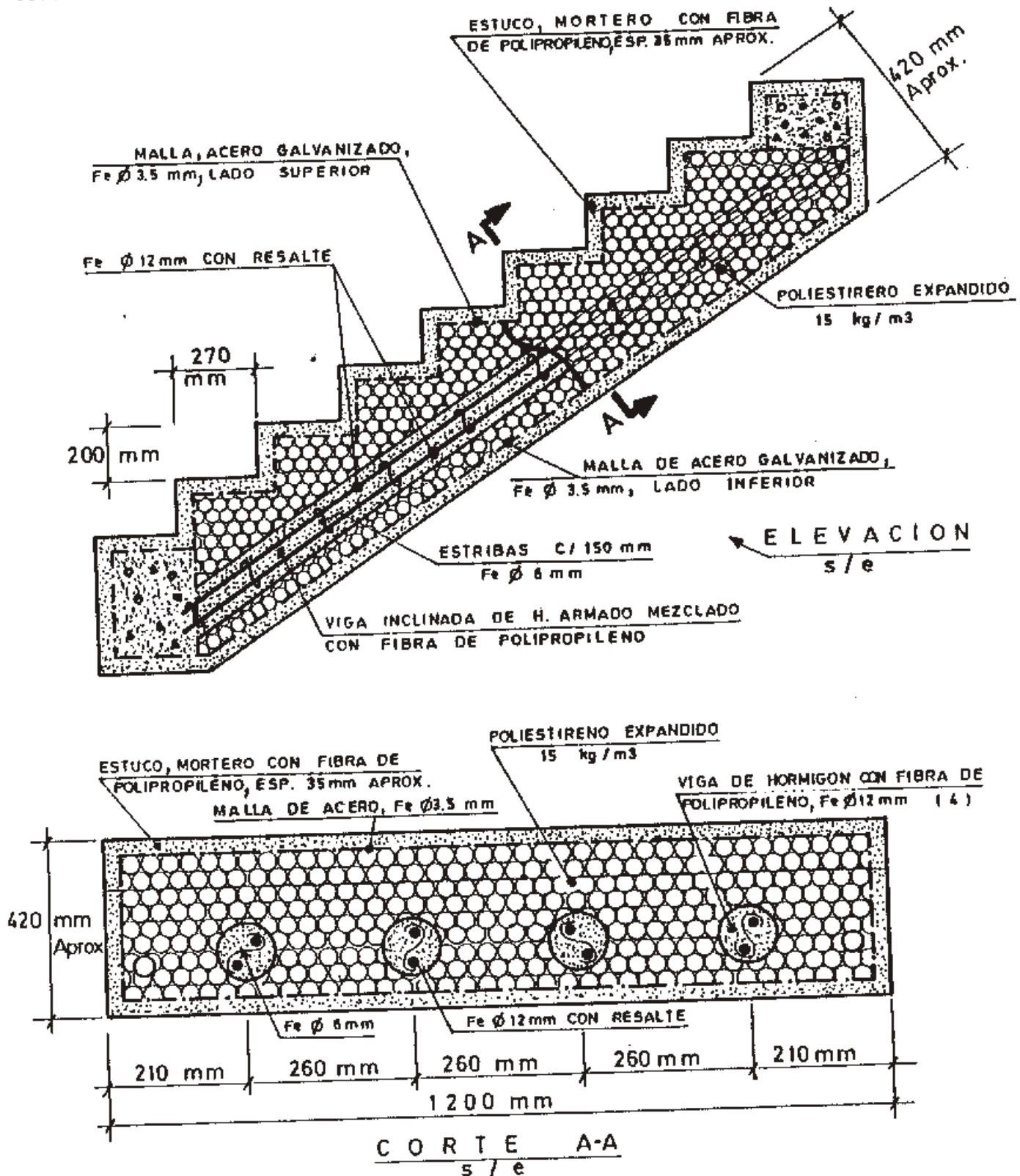
FIG. 1. ELEVACION Y CORTE DE LA ESCALERA.
